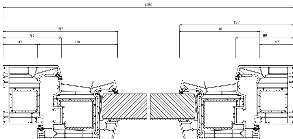
Schnitt S1(5:1)
